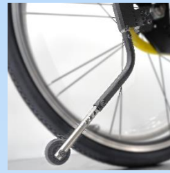
転倒防止ユニット
